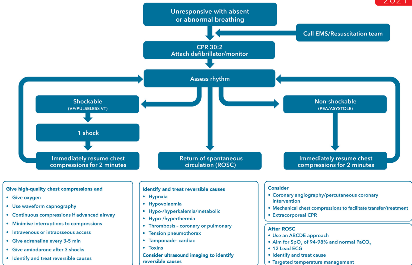
Fig. 8 – ALS algorithm.
